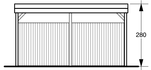
ZUIDWEST GEVEL
