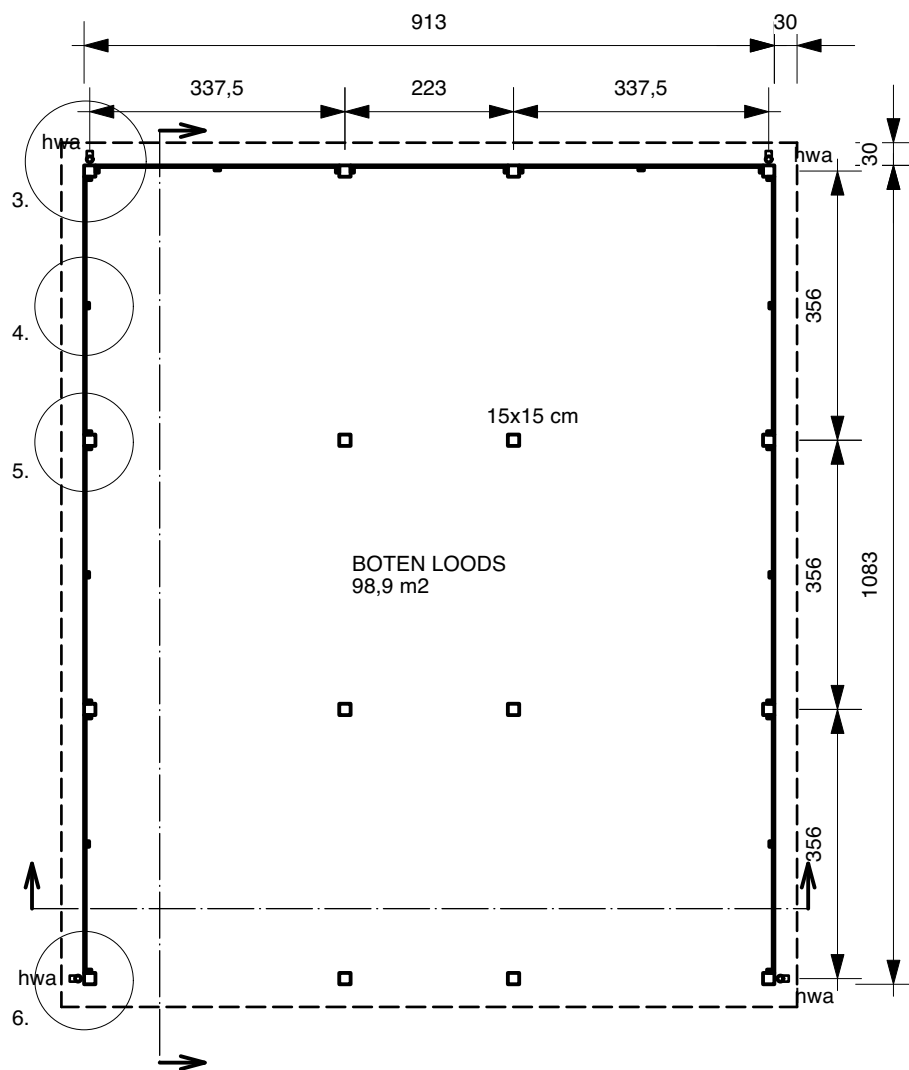
PLATTEGROND
