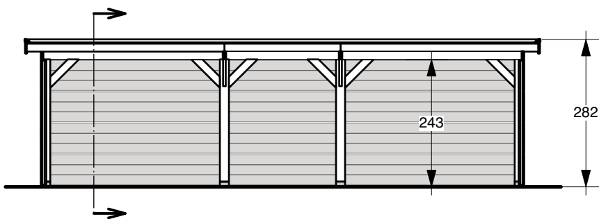
DWARSDOORSNEDE
